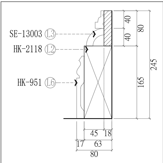
底座-線板側剖圖
