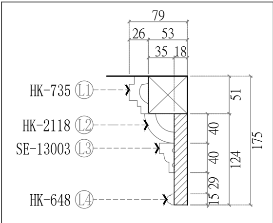
柱頭-線板側剖圖
