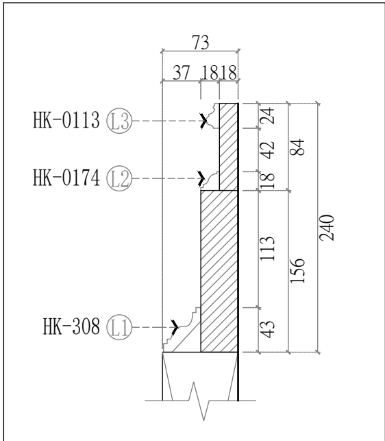
底座-線板側剖圖
