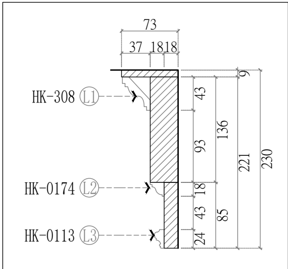
柱頭-線板側剖圖
