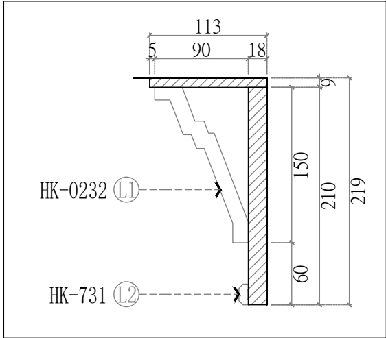
柱頭-線板側剖圖
