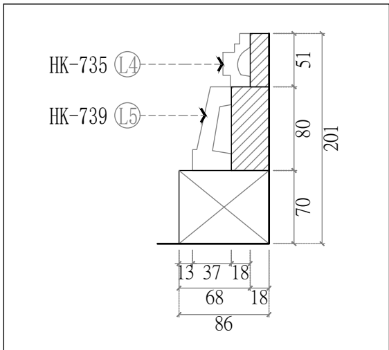
底座-線板側剖圖
