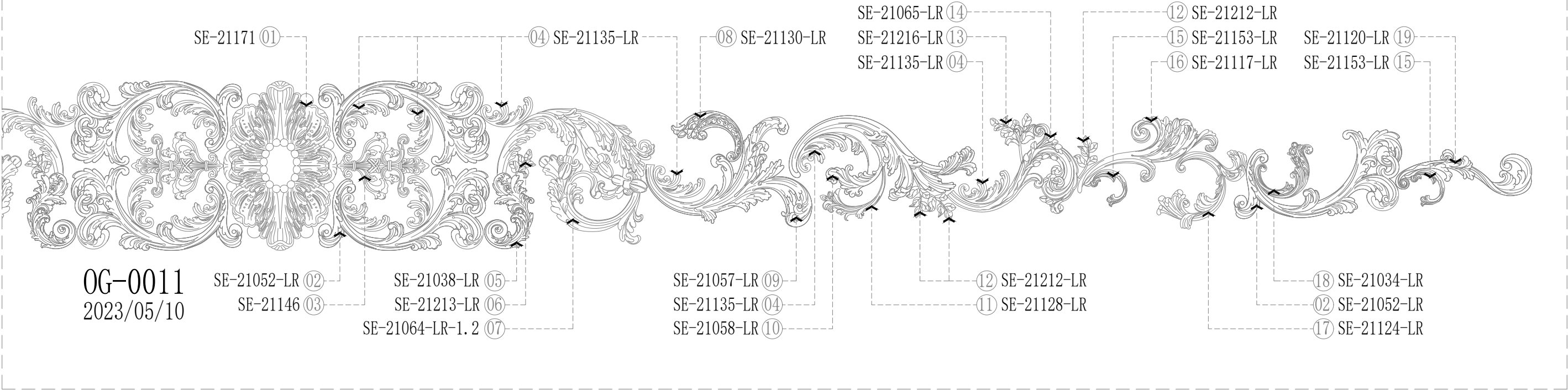
飾花詳圖
