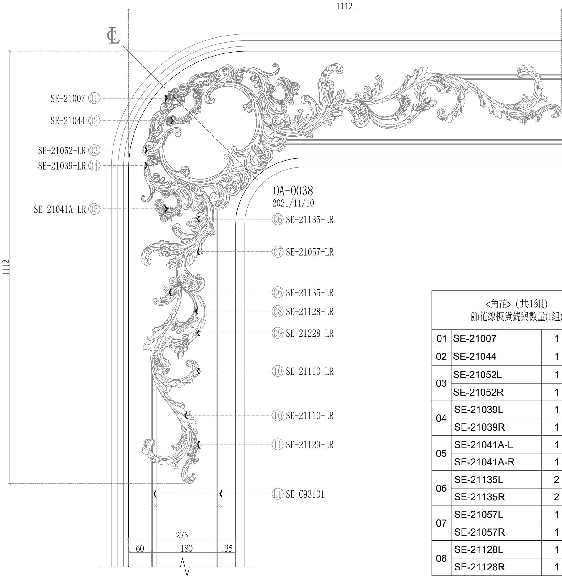
線板角花 弧面展開圖
