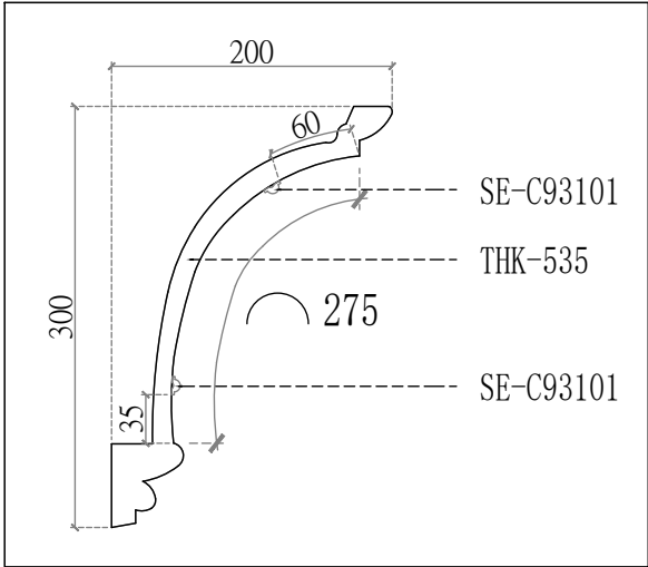
線板尺寸圖
