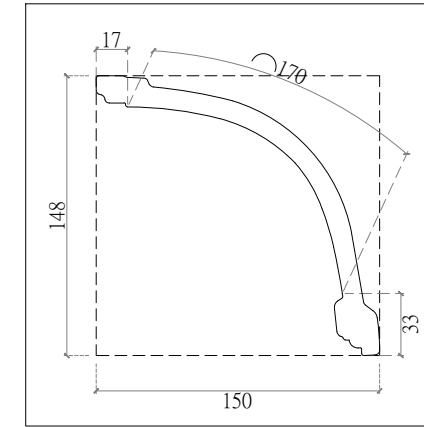
Ⓘ GM-0021 線板剖面圖
