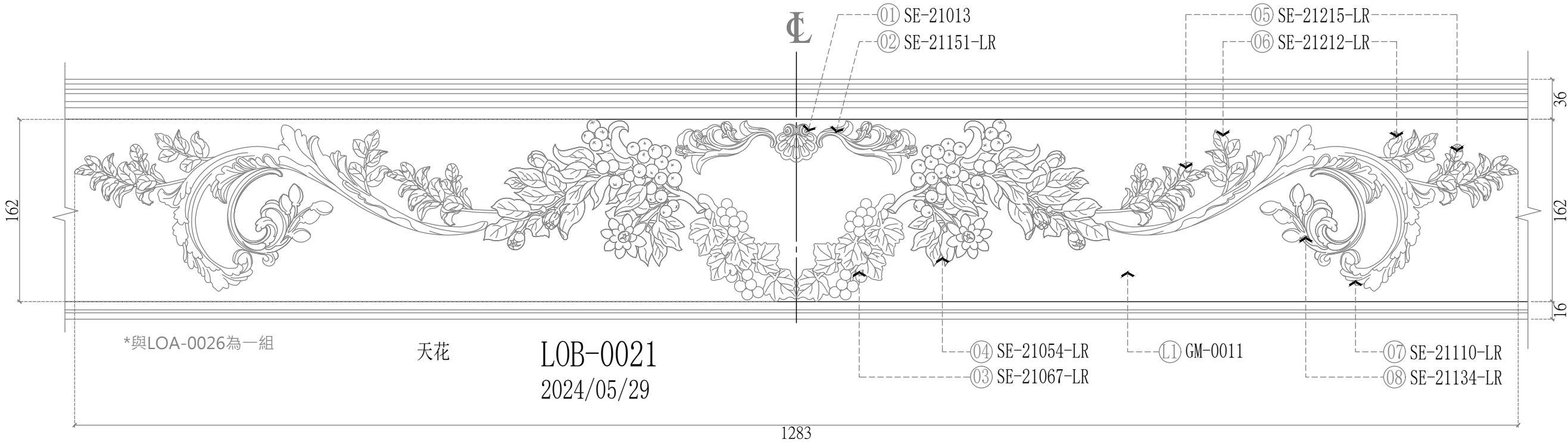
線板弧面展開圖
