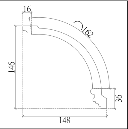
① GM-0011 線板剖面圖
