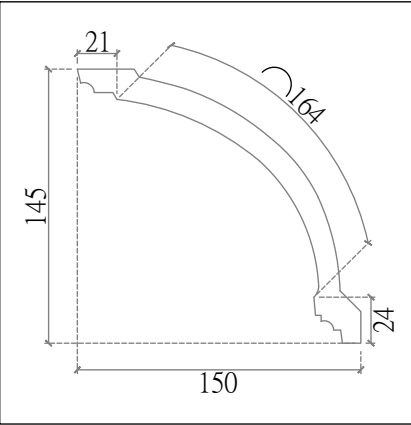
① GM-0021 線板剖面圖
