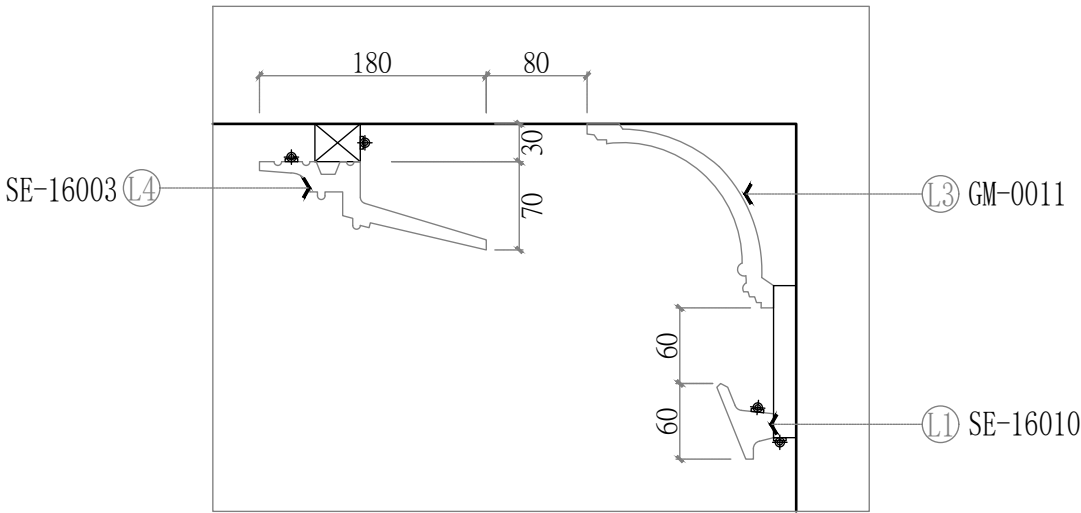
側剖 詳圖
