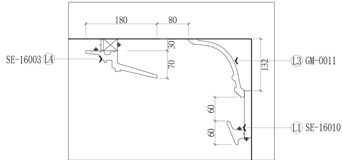
側剖 詳圖
