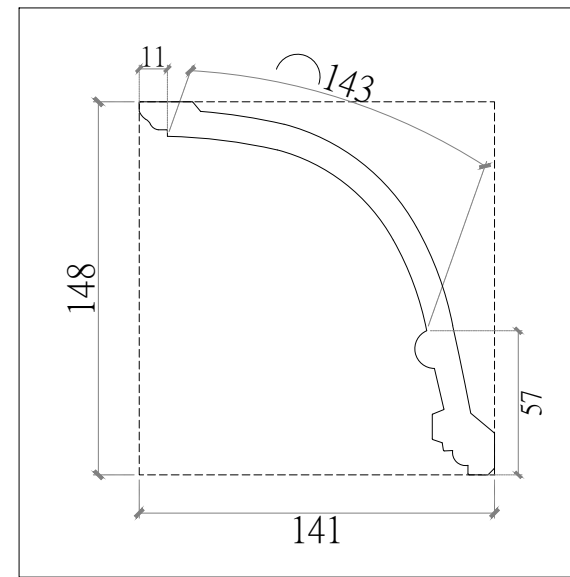
GM-0011 線板剖面圖
