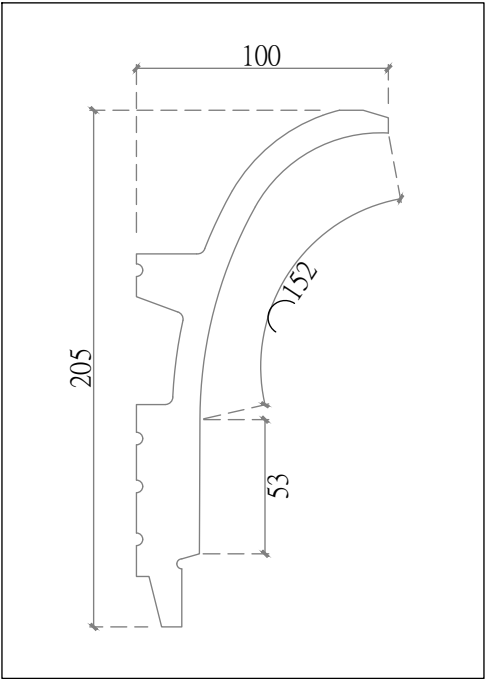
㊟ SE-16008 線板剖面圖
