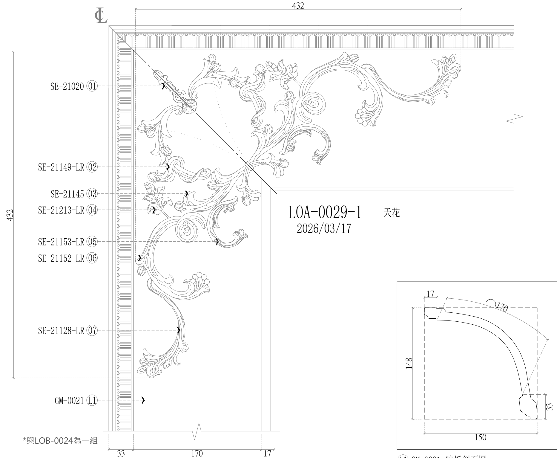
Ⓘ GM-0021 線板剖面圖
