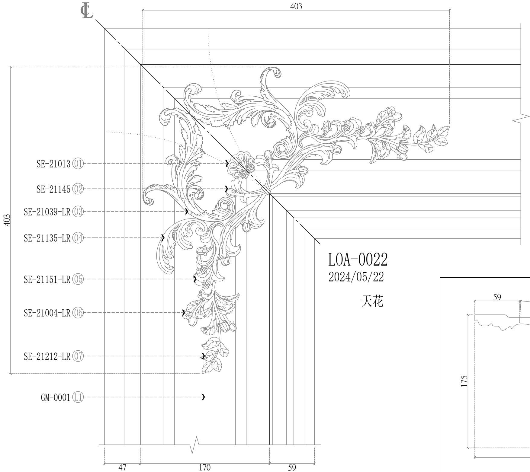
線板弧面展開圖
