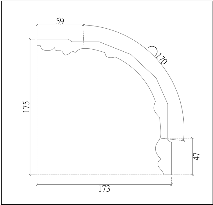
Ⓕ GM-0001 線板剖面圖
