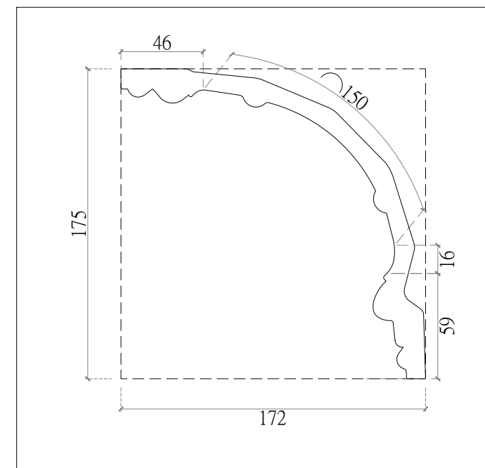
(L1) GM-0001 線板剖面圖
