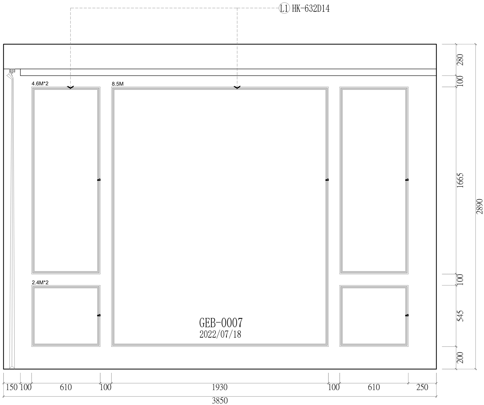
主卧室 床头背景 立面配置圖
