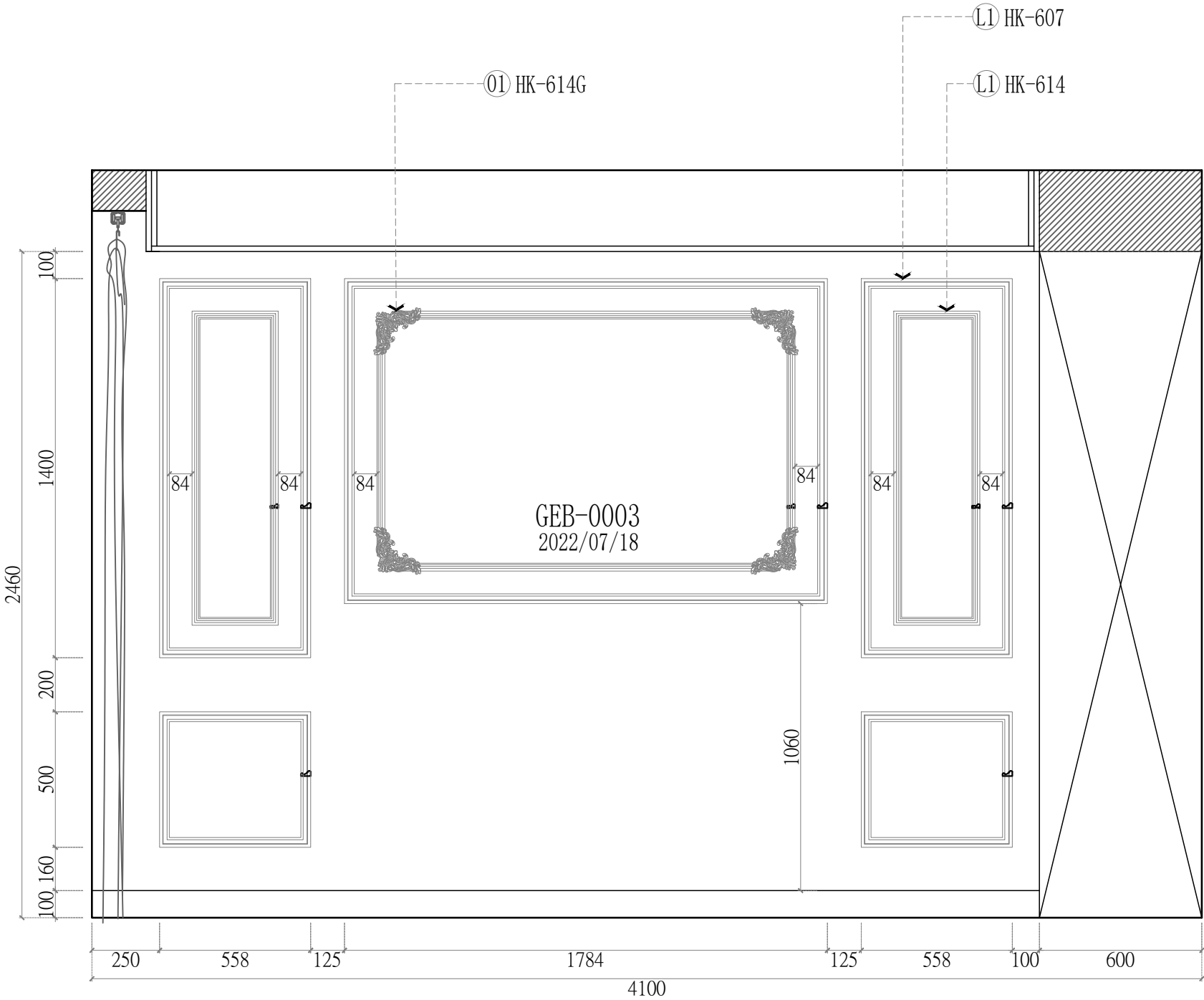
主卧 立面图
