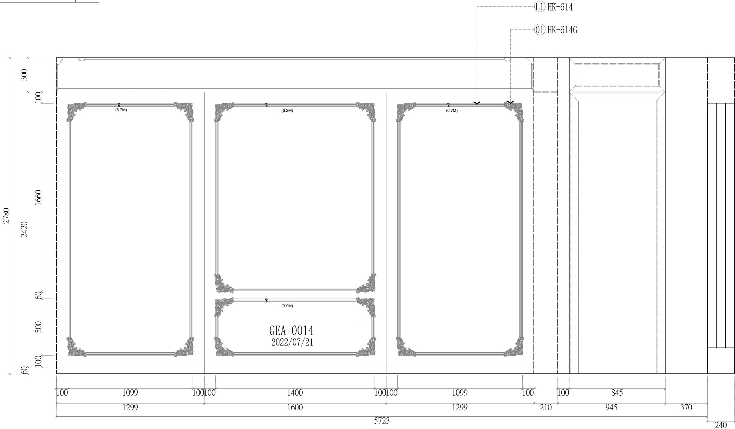
客廳 立面配置圖
