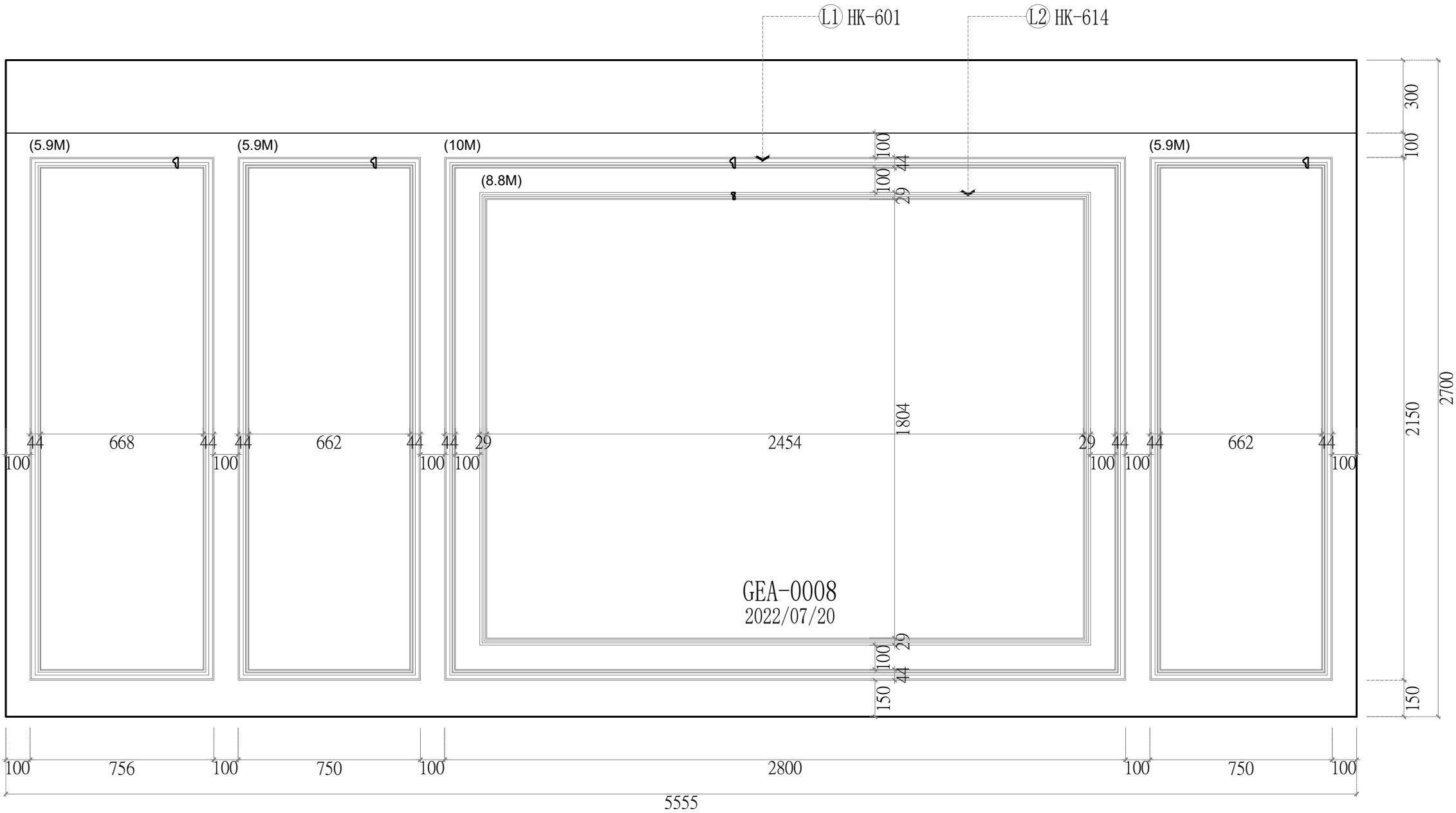
客廳 立面配置圖
