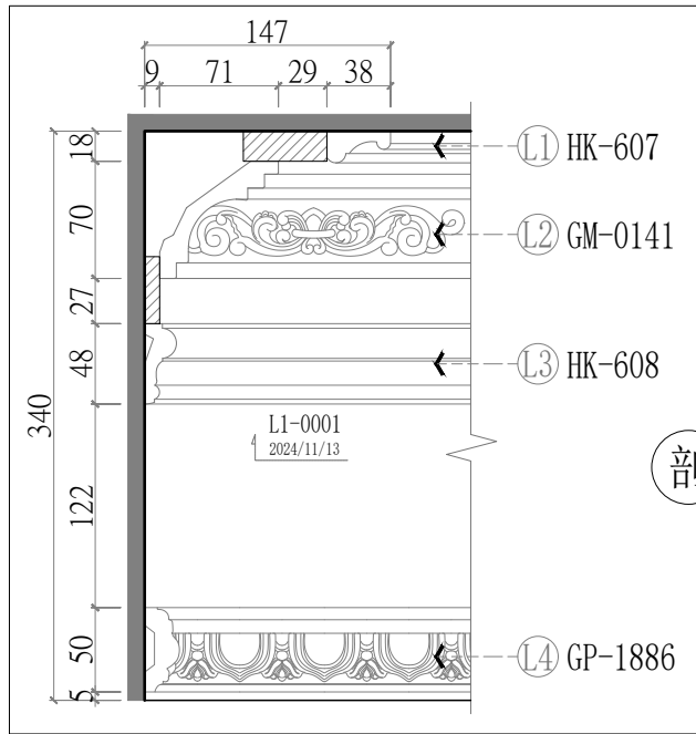
線板剖面圖
